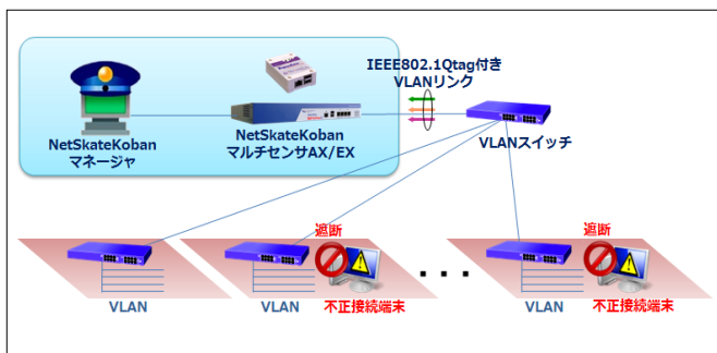
NetSkateKoban® マルチVLANセンサEX 監視構成イメージ
